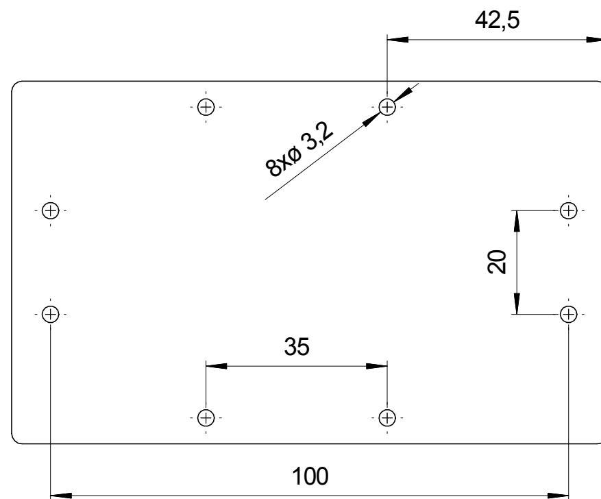
Vrchní deska
